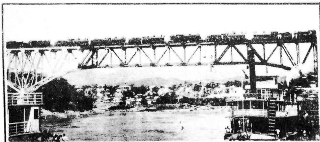
Prueba de resistencia, con nueve locomotoras, del magnífico puente construido sobre el Río Magdalena, y que se ha inaugurado en fecha próxima en la ciudad de Girardot, Colombia.
